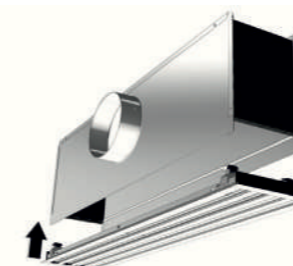
Insérer le diffuseur dans le plenum
