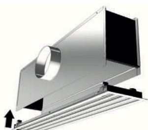
Insérer le diffuseur dans le plenum
