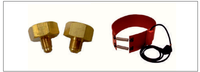
Raccord bouteille inversé R32 16244
